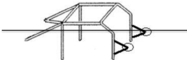
—Diagram 8.3(6)(d) — forward reinforcement —
